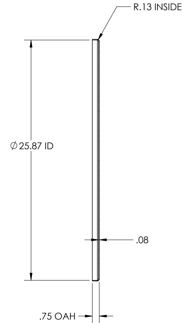
SECTION A-A SCALE 1 : 6
